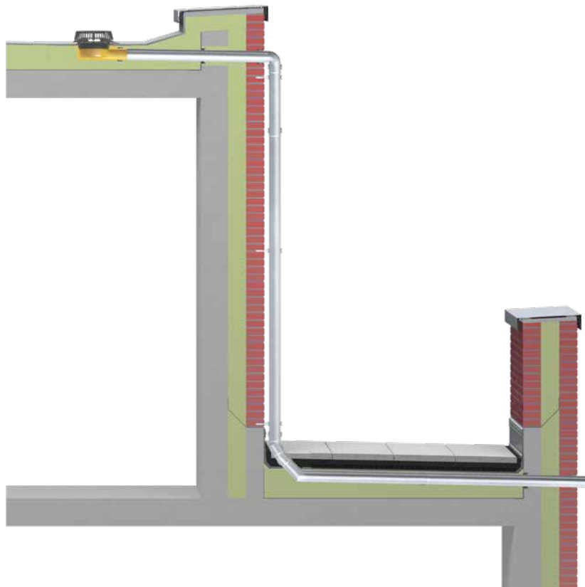
Bild 1: Beispiel einer normenkonformen „Kaskadenentwässerung“ der Sita Bauelemente GmbH
